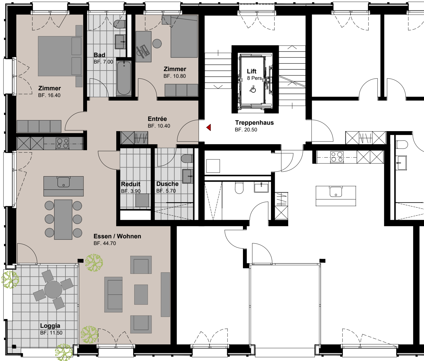
Obergeschoss
